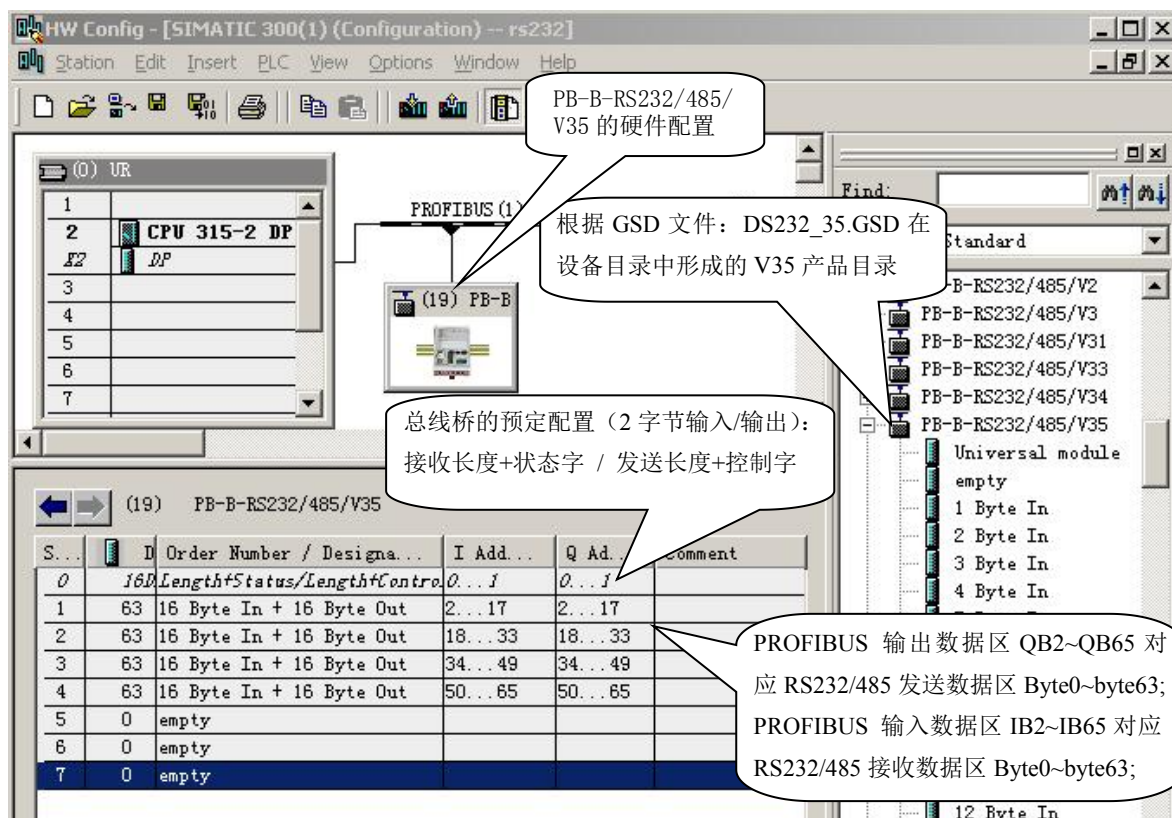
图 3-9 总线桥在 S7-300 主站中 PROFIBUS I/O 配置与 RS232/485 通信数据区的对应
