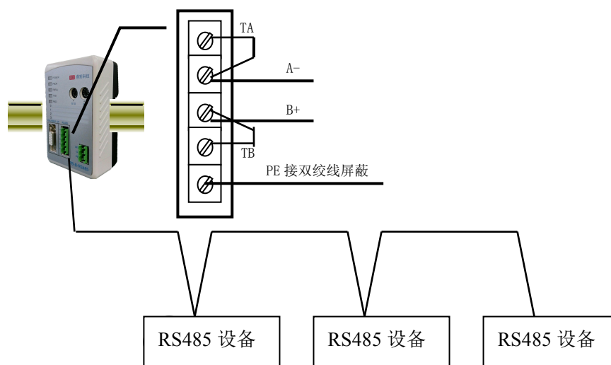
图 2-11 PB-B-RS485/V3x 位于 RS485 总线终端时端子接线方法
