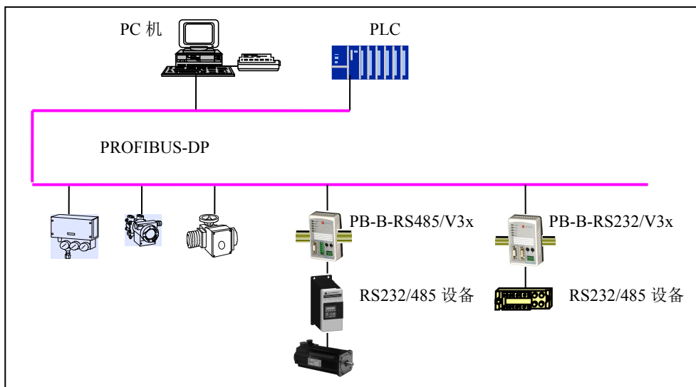
图 3-3 PLC 为主站的 PROFIBUS 系统中使用总线桥将设备连接到 PROFIBUS-DP 上
