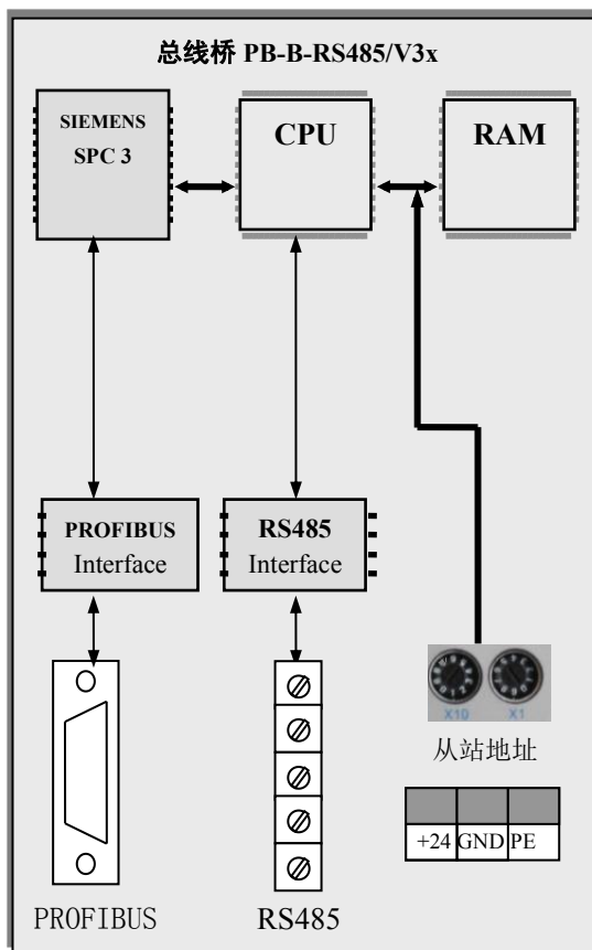
图 3-2 PB-B-RS485/V3x 硬件结构
