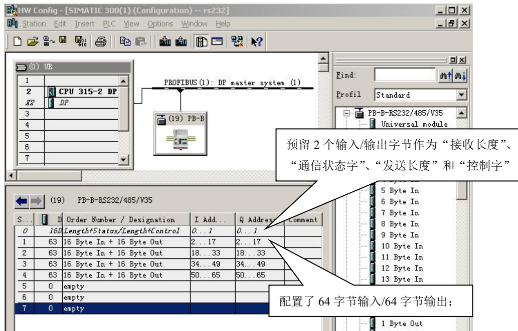
图 3-6 一个 PROFIBUS 总线桥输入/输出配置的实例
