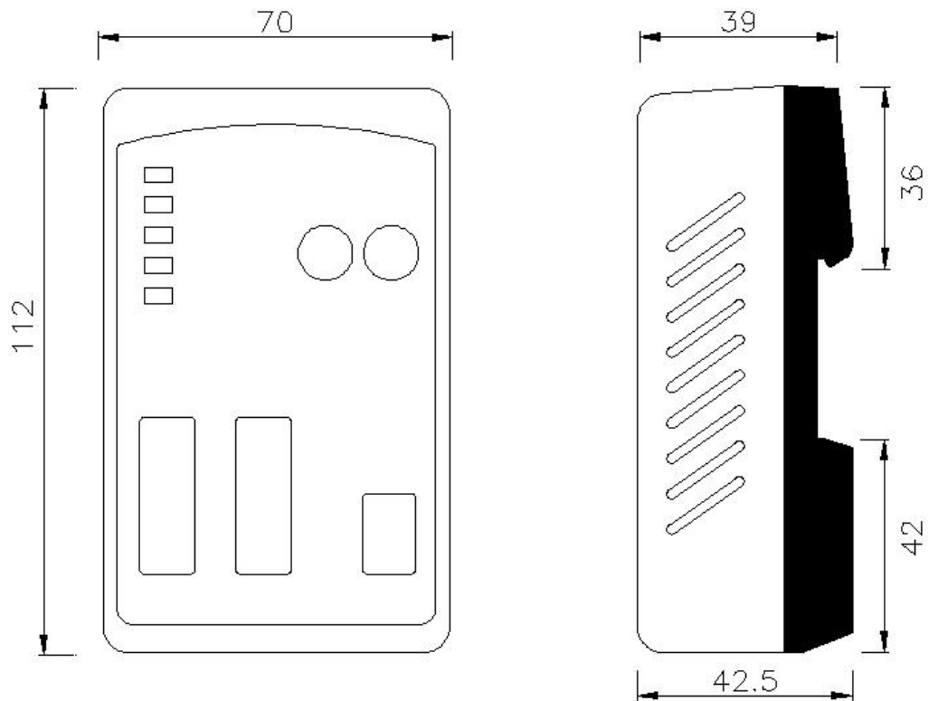
图 2-4 产品外形尺寸图
