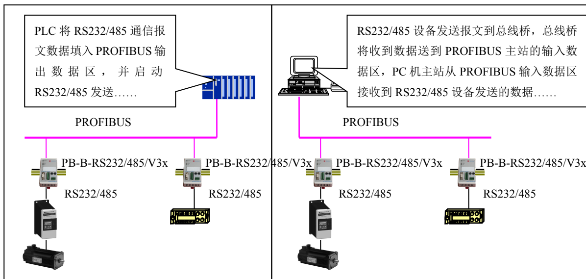
图 3-5 接收/发送过程
