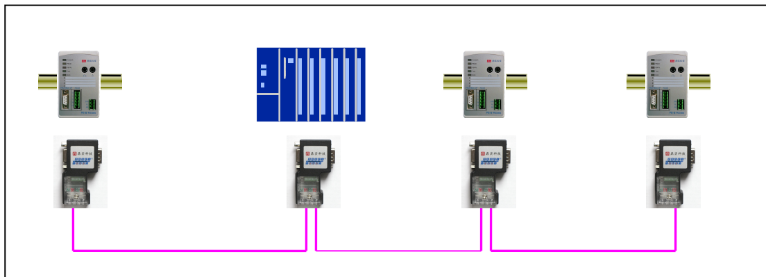
图 2-5 PROFIBUS 接口采用 9 针 D 形插座 (孔), 建议用户使用标准 PROFIBUS 插头及电缆
