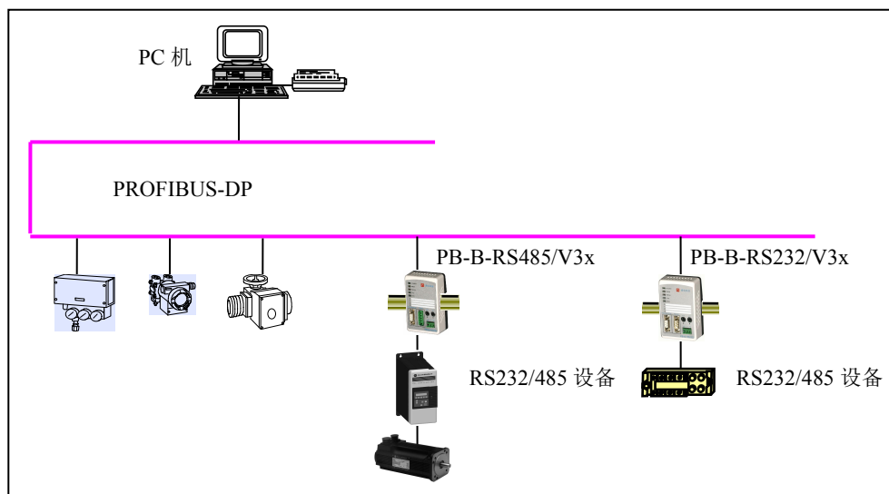
图 3-4 基于 PC 的现场总线控制系统使用总线桥将设备连接到 PROFIBUS-DP 上
