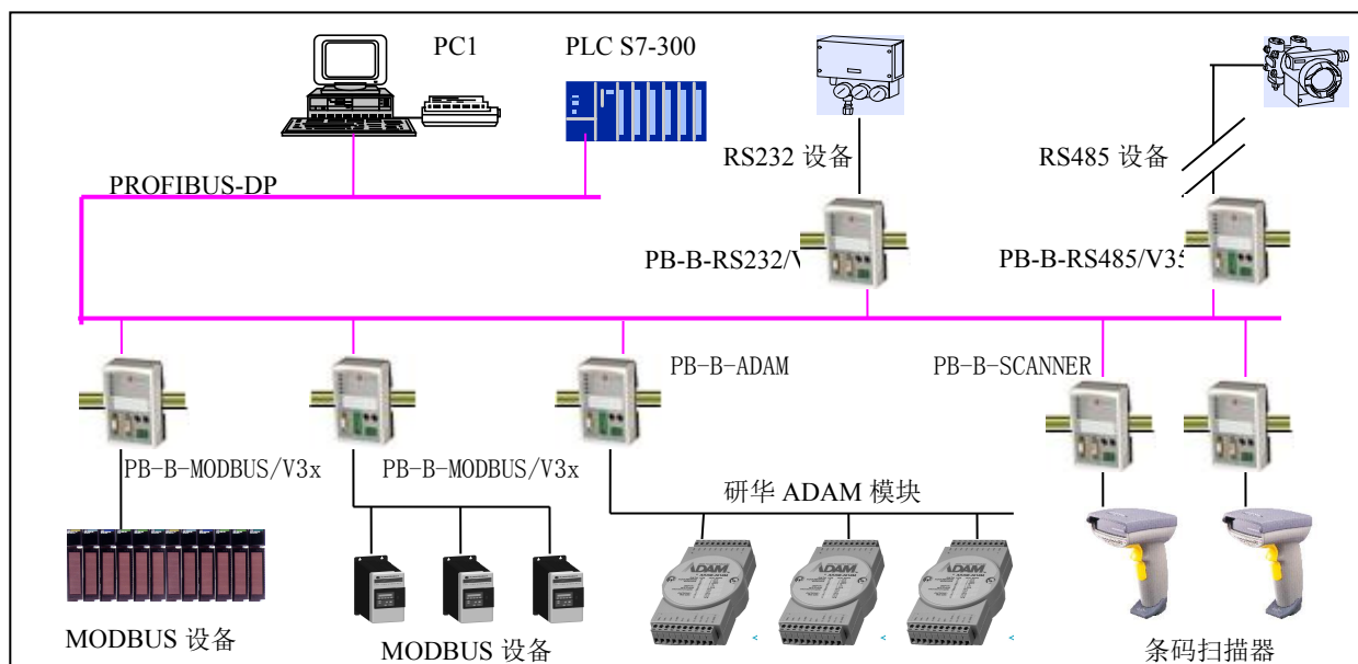
图 1-1 具有不同通信协议的的设备与 PROFIBUS 总线桥的连接
