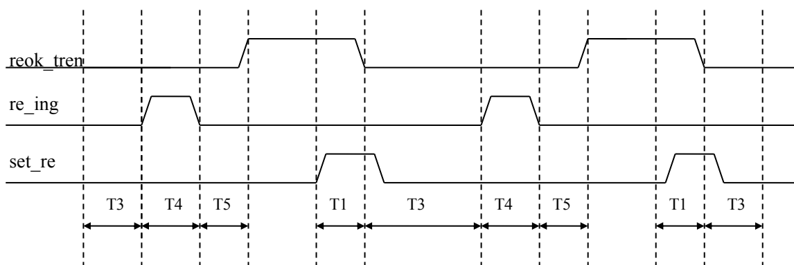
图 3-24 典型的“收→收→”过程时序图
