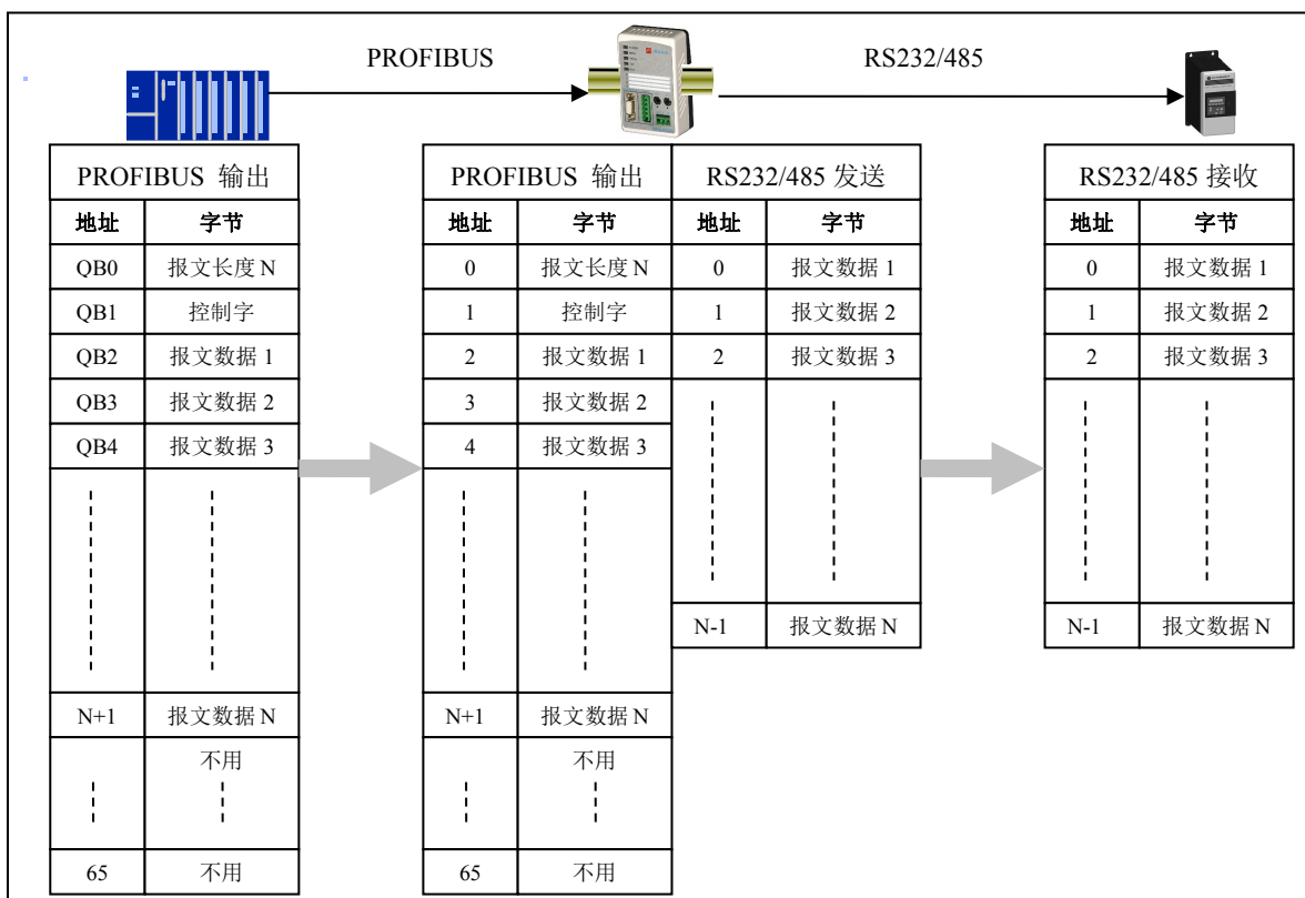
图 3-11 PROFIBUS 主站、接口、现场设备之间的报文格式
